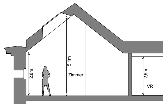
Schnitt B
