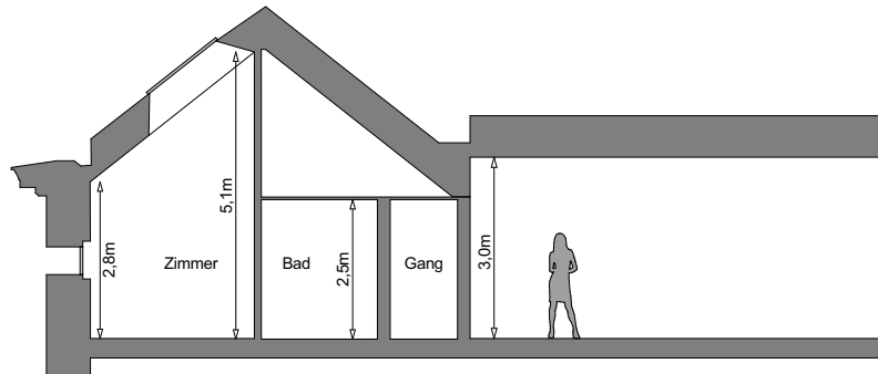
Schnitt B
