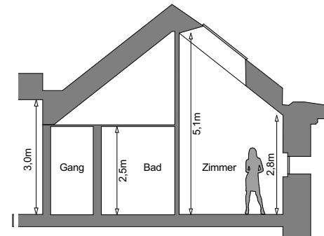
Schnitt B
